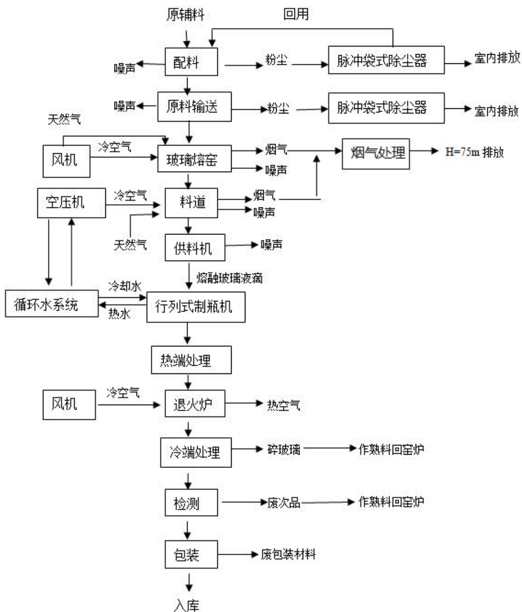
图 2-1 生产工艺流程图
