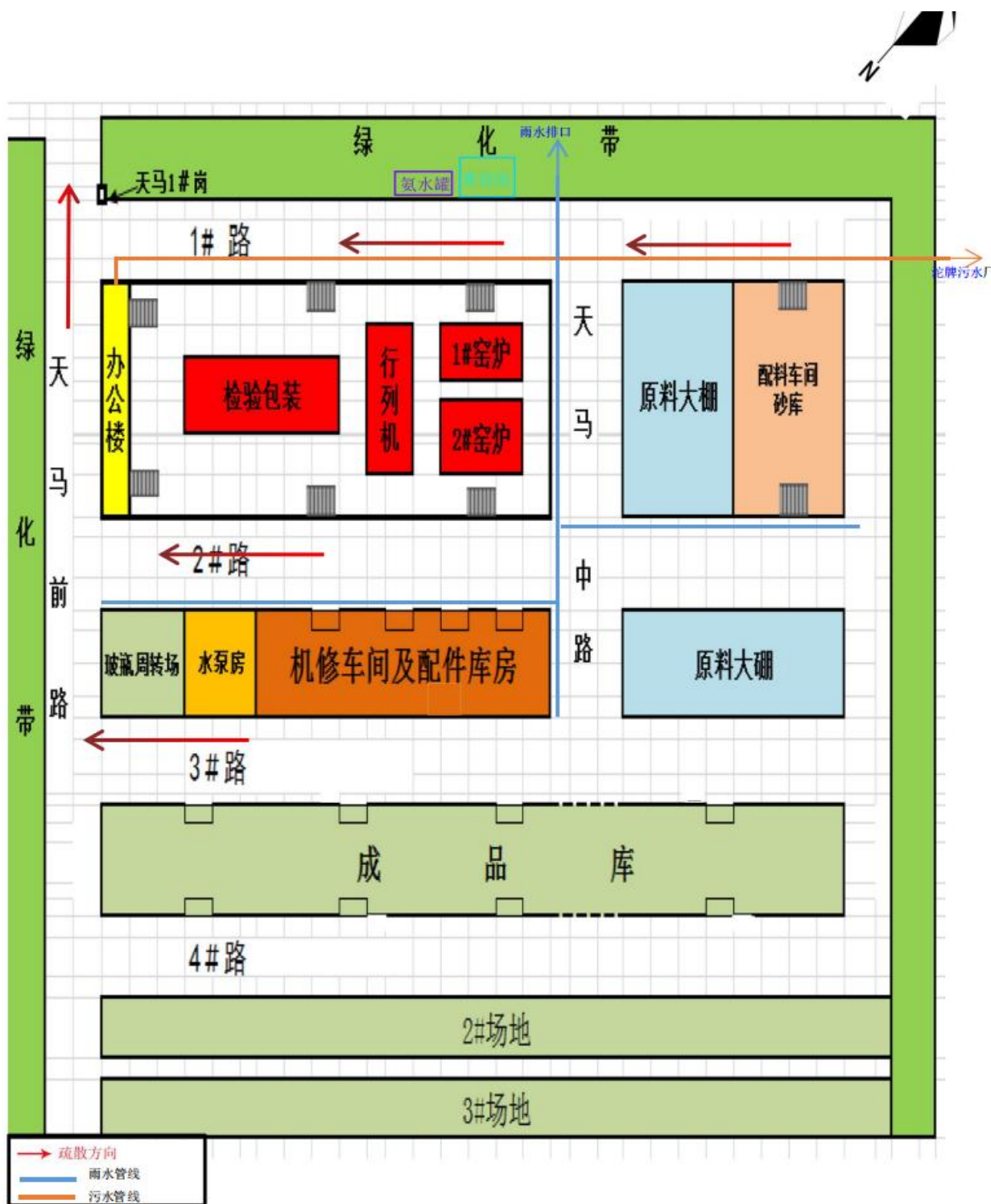
附图 6 项目雨污分流图
